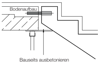
Auflager mit Gewindestangen (ohne Schallschutz)
