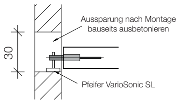
Zwischenaufleger mit Pfeifer VarioSonic SL ohne Schaumstoffbox (ohne Schallschutz)
