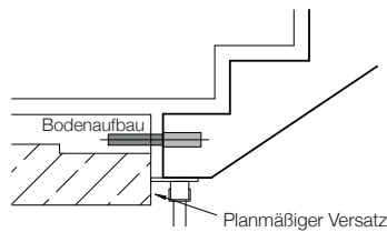
Auflager mit Gewindestangen (ohne Schallschutz)
