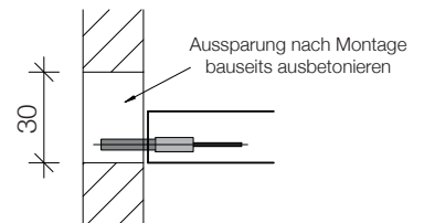
Zwischenaufleger mit Gewindestangen (ohne Schallschutz)
