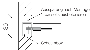
Zwischenaufleger mit Pfeifer VarioSonic SL mit Schaumstoffbox (mit Schallschutz)
